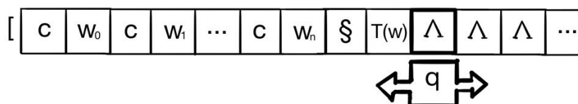
рис. 3.3 лента в состоянии останова
