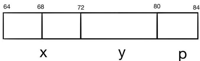
рис. 9.7 расположение переменных в памяти
