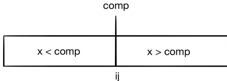
рис. 19.10 массив по завершении внешнего цикла
