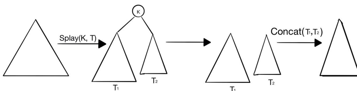
рис. 23.8 операция удаления
