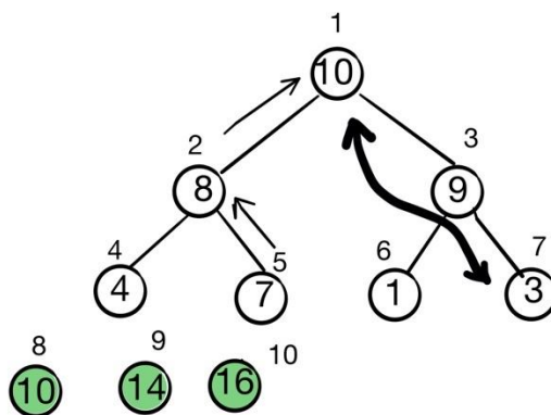
рис. 24.8
