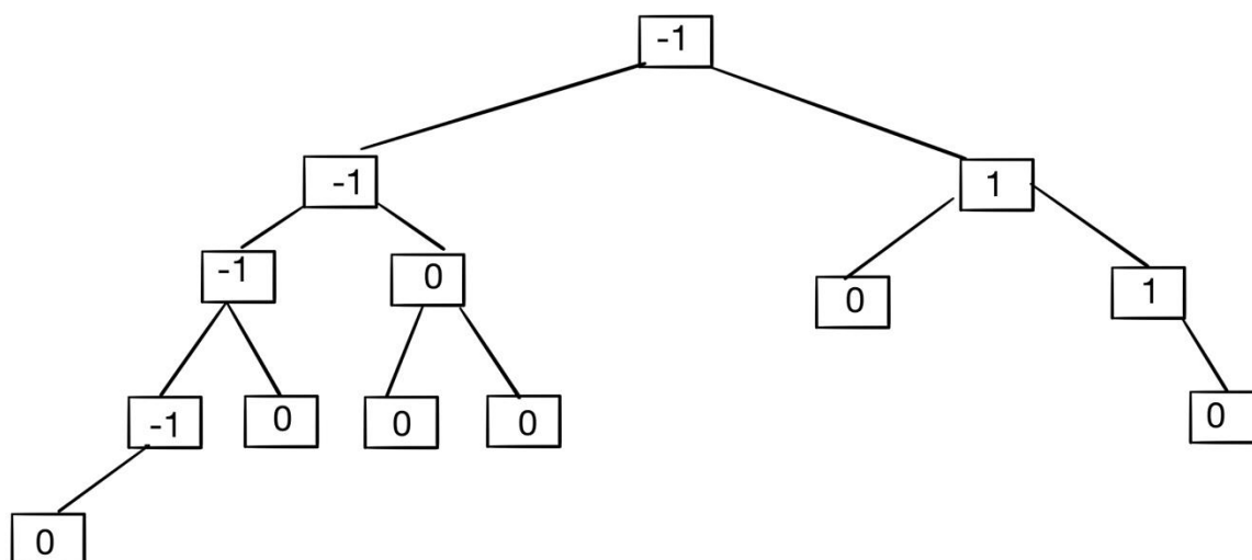
рис. 22.2 АВЛ-дерево
