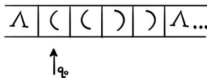
рис. 2.1 Начальное состояние
