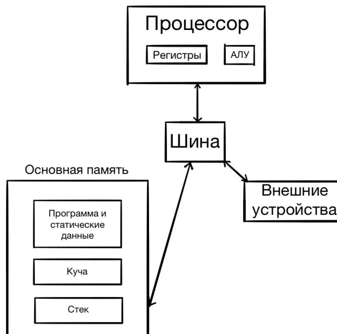
рис. 4.1 архитектура машины Си
