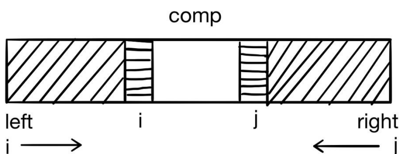
рис. 19.9 разделение массива
