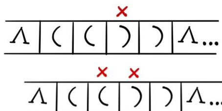
рис. 2.2 Маркеры
