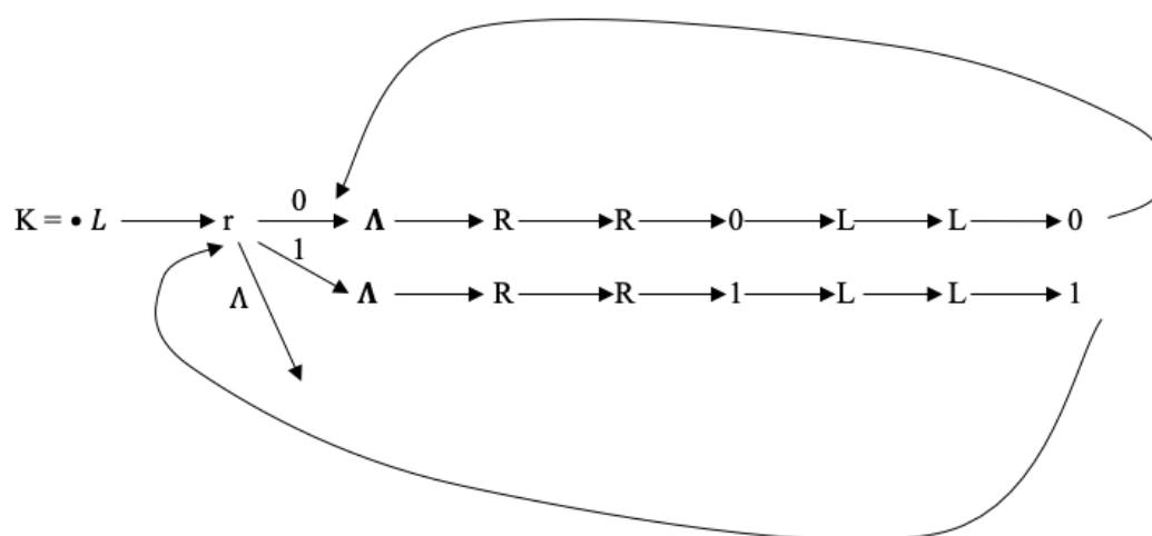
рис. 2.13 диаграмма К
