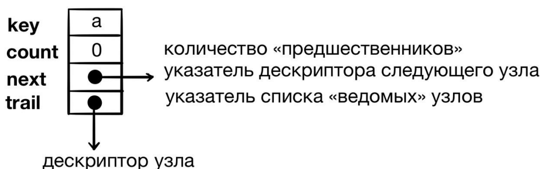
рис. 18.7 дескриптор узла
