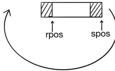
рис. 17.4 «закольцованная» очередь
