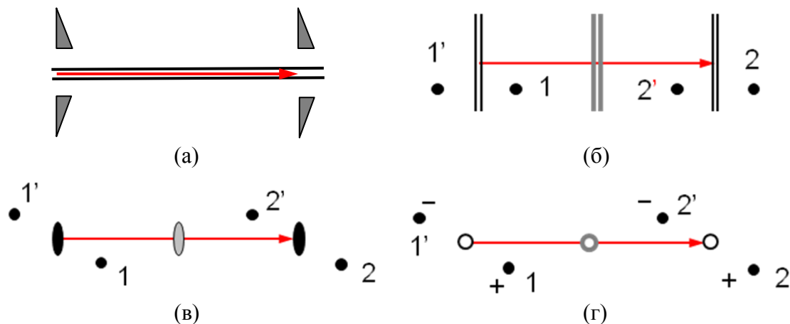
Рисунок 2.19. Взаимодействие трансляций \mathbf{t} (показаны красными стрелками) с элементами симметрии 2-го порядка: (а) параллельными трансляции (новых элементов не возникает), (б, в) перпендикулярными к трансляции, (г) с центром инверсии.
