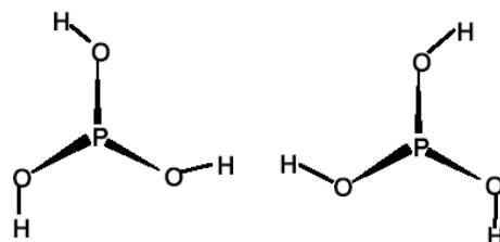
Рис. 1.1. Хиральная молекула \text{H}_3\text{PO}_3 , точечная группа C_3 (см. далее)
