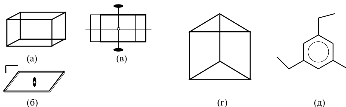
Рис. 1.9 Вид прямого параллелепипеда (а) и его проекции на основание (б) и боковую грань (в); (г) правильная треугольная призма, (д) молекула C_6H_3(OH)_3 .
